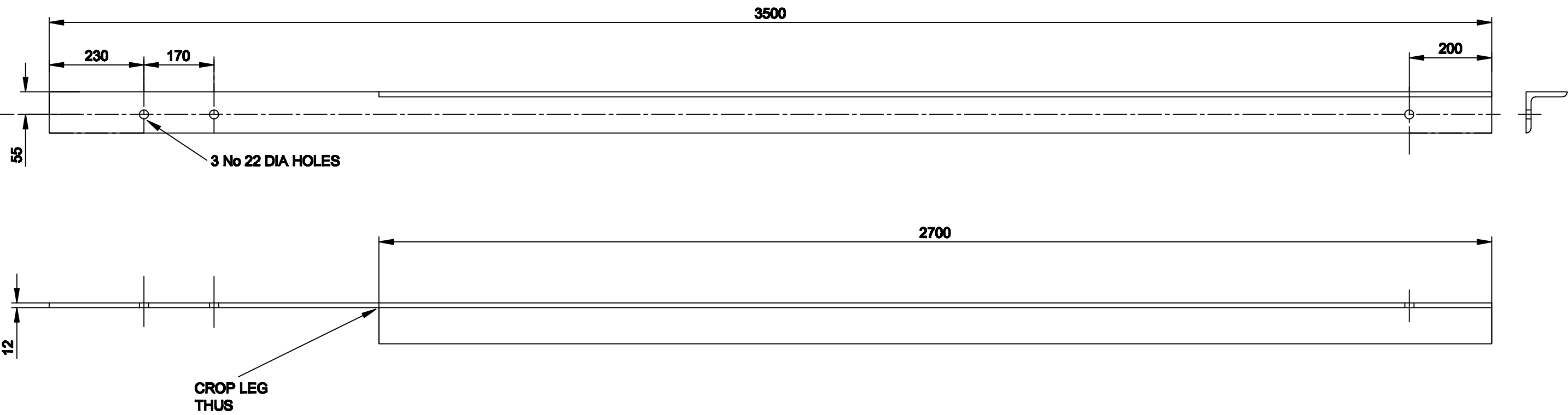
ITEM 9 100 x 100 x 12 ANGLE - 3500 LONG SCALE 1 : 10
